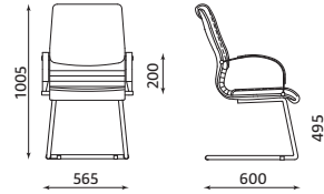
ARTUS-LB CF
