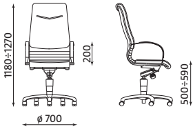
ARTUS MPD170
